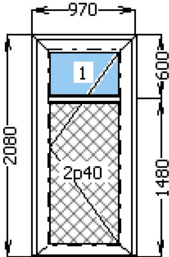
Рис.2.1 Креслення металопластикових дверей
