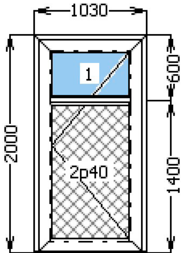
Рис.2.2 Креслення металопластикових дверей
