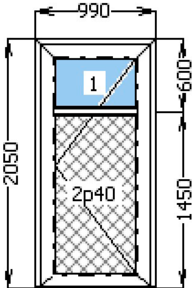
Рис.2.1 Креслення металопластикових дверей
