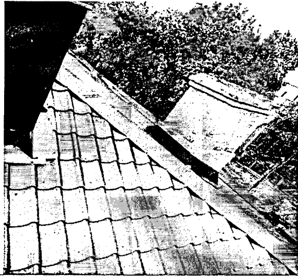
Опис фото №6 улаштування металочерпиці та сніготримачів
