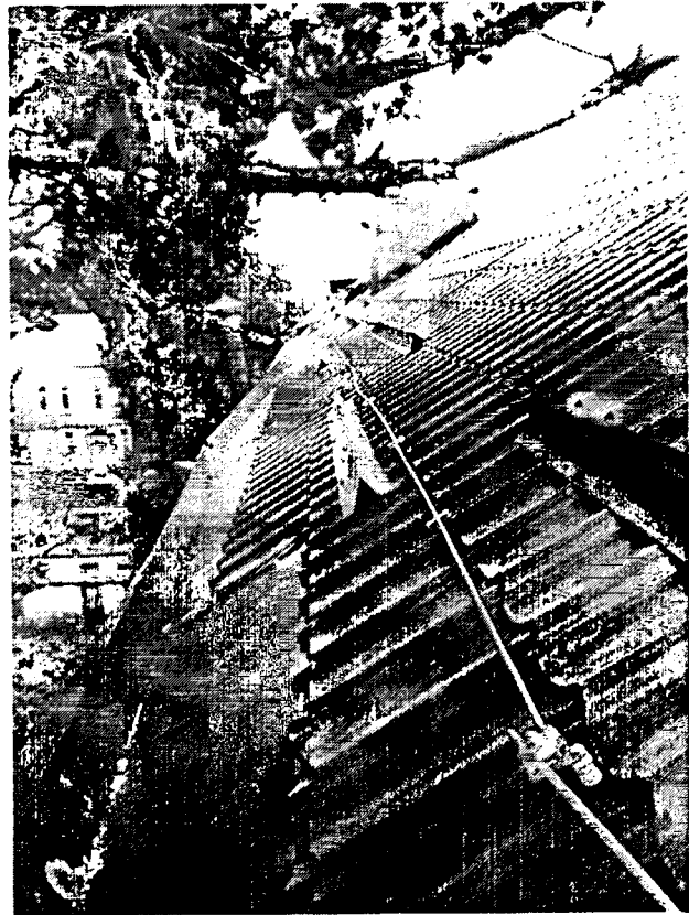
Опис фото №11 улаштування блискавкозахиста та сніготримачів
