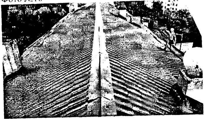
Опис фото № 16 улаштування коньків, готова покрівля
