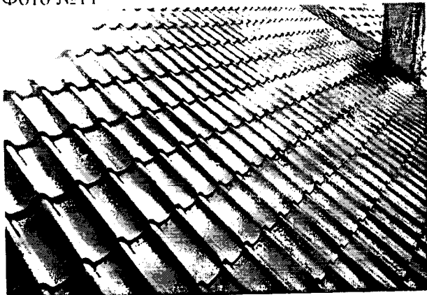
Опис фото №11 улаштування металочерепиці
