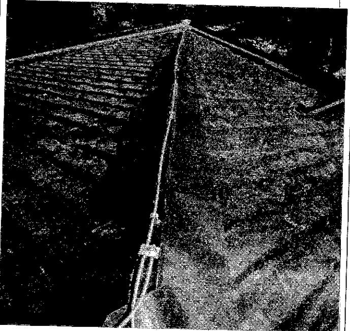
Опис фото №18 Влаштування блискавкозахисту
