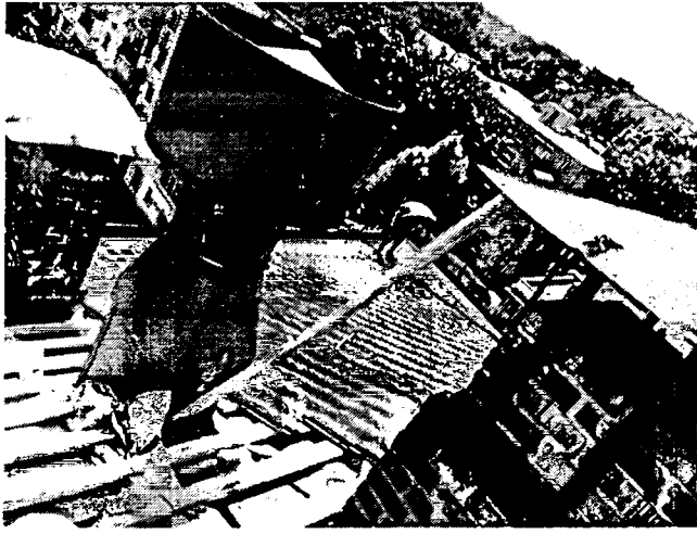
Опис фото № улаштування плівки «гідробар'єр», обрешетування та металочерепиці
