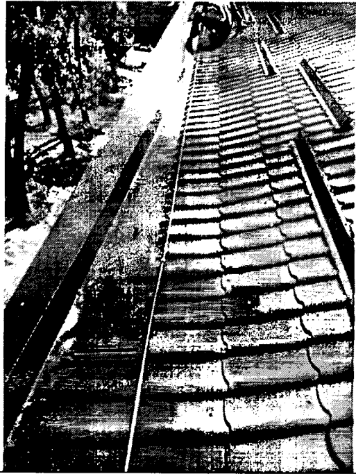
Опис фото №12 улаштування металочерепиці, сніготримачів та блискавкозахиста
